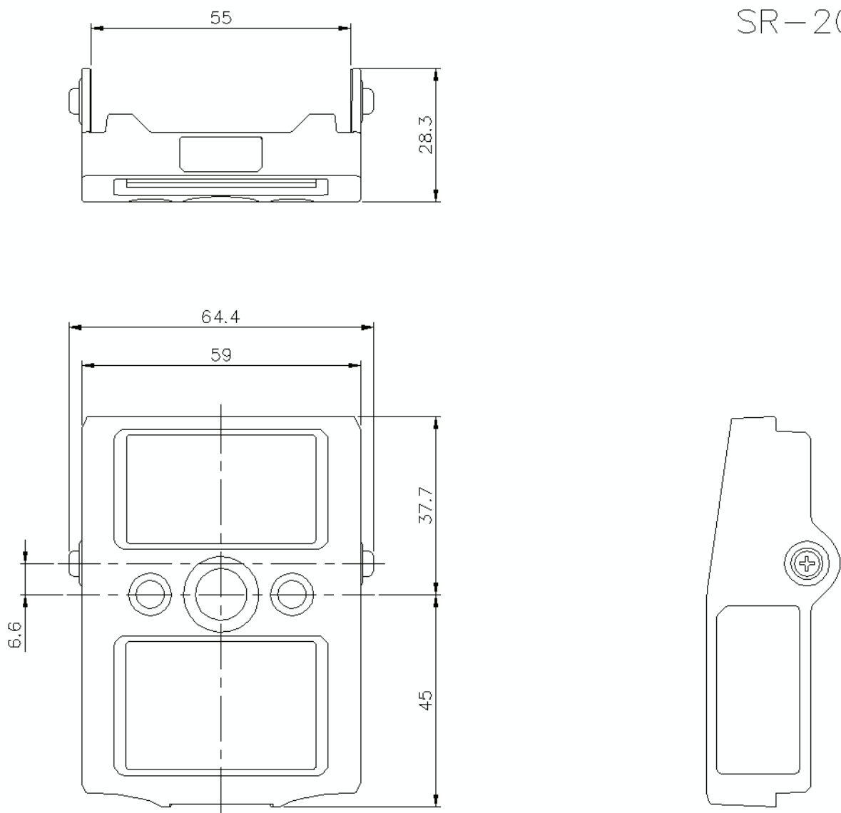
sr-20ah_dimension_01.gif
